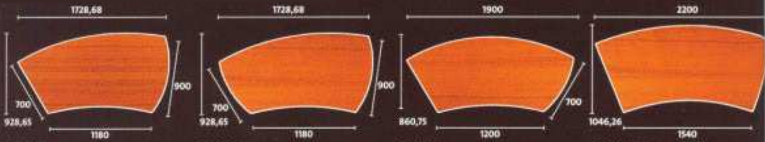
Tischplatte Tabletop Tischplatte Tabletop Tischplatte Tabletop Tischplatte, Bogenmaß 43° Tabletop, angle 43°
